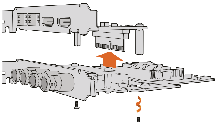
夹层卡的移除和安装很简单
