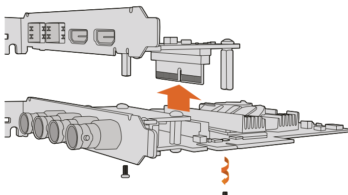
Mezzanin-Karten lassen sich einfach entfernen und anbringen
