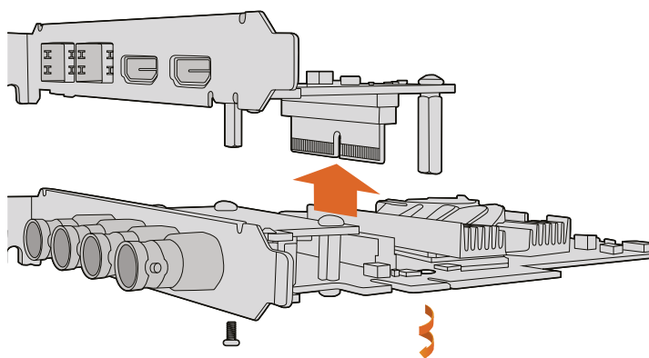
Les cartes mezzanine peuvent être facilement retirées et attachées
