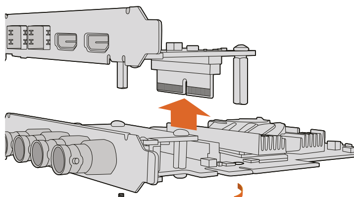
メザニンカードは簡単に取り外し、取り付けが可能
