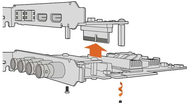
Mezzanine kartlar kolaylıkla çıkarılıp takılabilir
