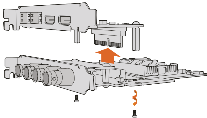
메자닌 카드는 쉽게 제거 및 설치할 수 있습니다.
