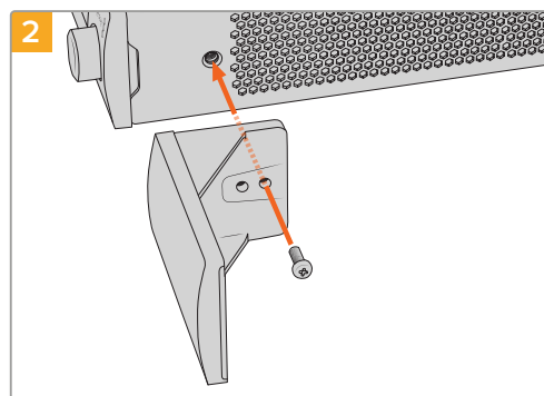
Выверните заглушку и закрепите ее с помощью прилагаемого 9-мм винта M3
