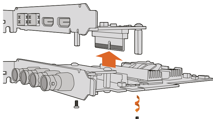
Мезонинные платы допускают легкий монтаж и демонтаж
