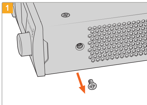
Entfernen Sie die 5mm-M3-Schraube nahe der Frontblende
